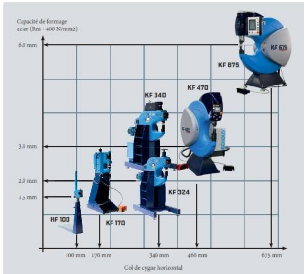
Col de cygne horizontal / Sbraccio orizzontale
