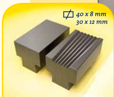
1115 (LH 34 / 40) 130 x 80 mm 2115 (LH 50 / 60) 130 x 80 mm
