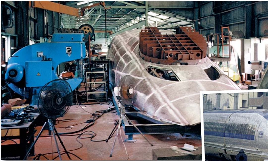
Formage de pièces de carrosserie du train express SHINKANSEN (Japon) sur des machines Kraftformer ECKOLD.
